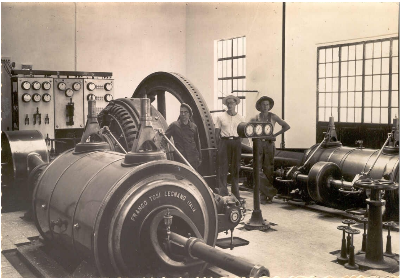
Generadores de la fábrica. Marca FRANCO TOSI LEGNANO, ITALIA.
